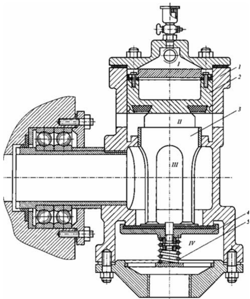
Рис. 5.24. Схема воздухоподводящей головки
